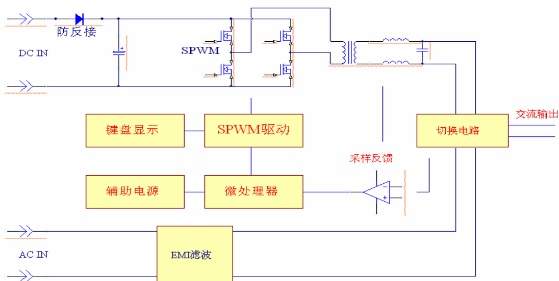
图 1：逆变电源功能框图
